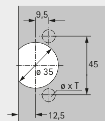
Boorbeeld 45 x 9,5 mm
