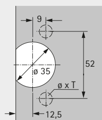
Boorbeeld 52 x 9 mm
