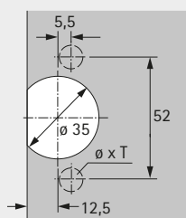
Boorbeeld 52 x 5,5 mm
